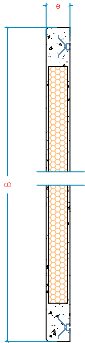
SECCION
