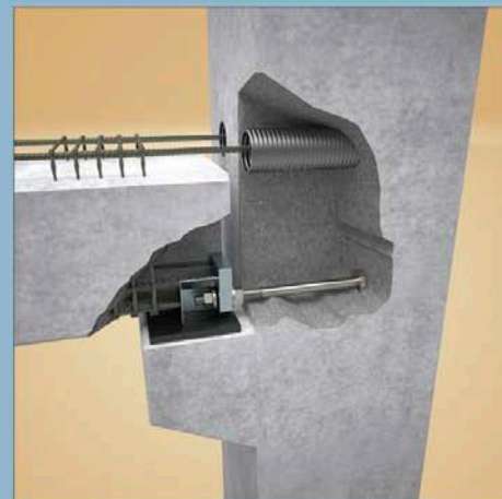
CONEXION HIPERESTATICA
